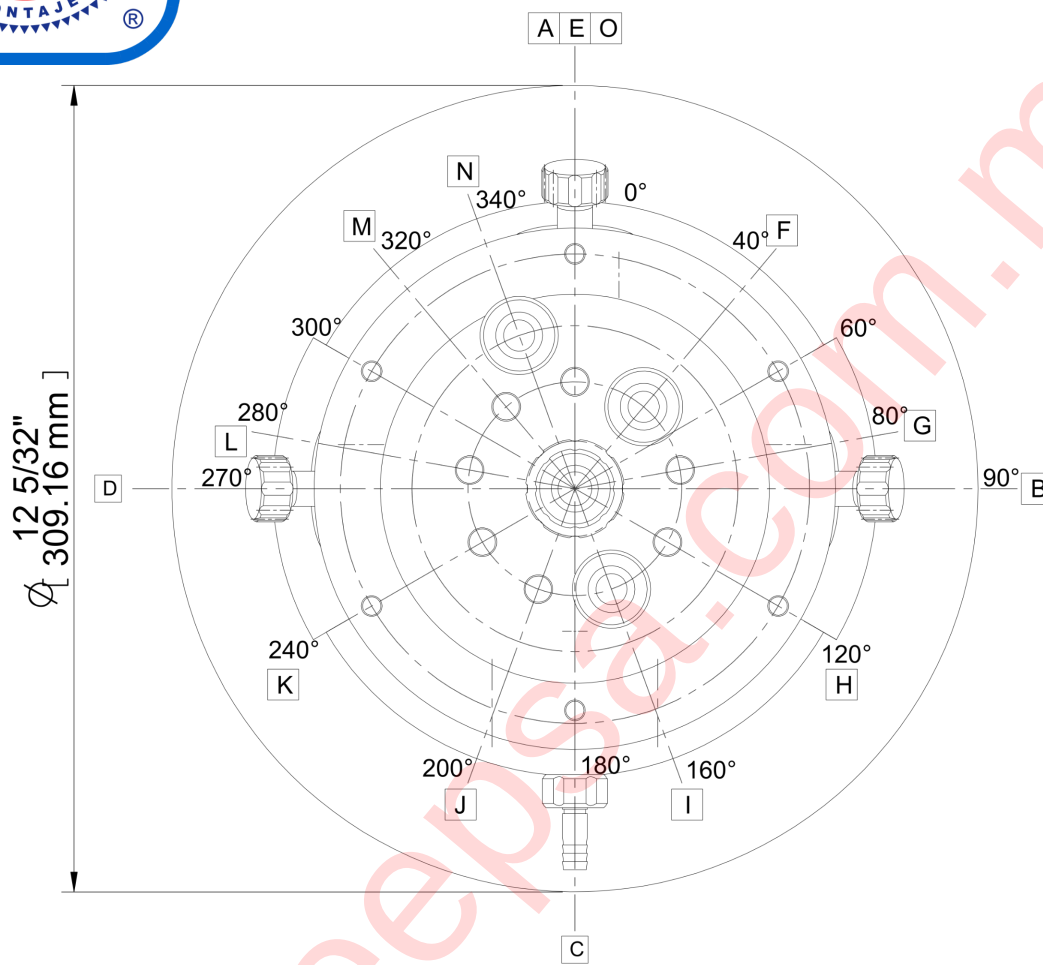
VISTA SUPERIOR
